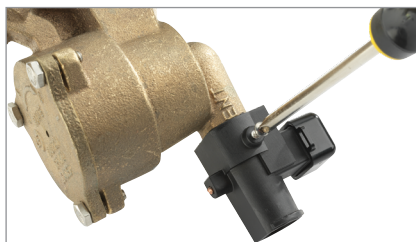
2. Utilice el destornillador Phillips n.º 2 para fijar el sensor a la válvula de alivio.
