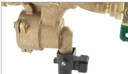
3. Veillez à ce que l'interface du capteur soit orientée dans la même direction que la flèche de débit de la vanne.
