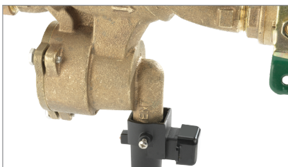
3. Asegúrese de que la interfaz del sensor apunte en la misma dirección que la flecha de flujo de la válvula.
